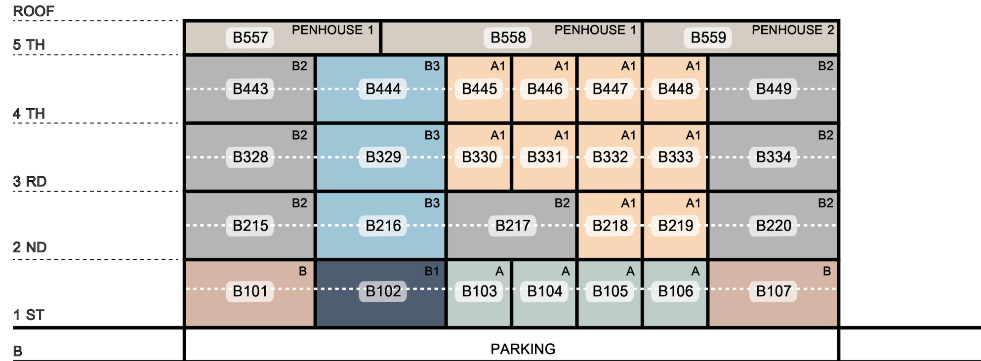
SECTION 01
